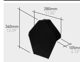
Q147*K | End cap 45° klinker
