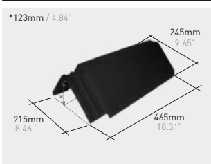
Q145*K | Ridge 45° klinker
