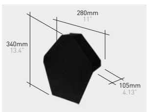
Q147*K | End cap 45° klinker
