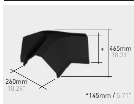
Q146*K | 45° 3 way ridge klinker
