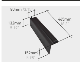
Q115*K | Innova/Vienna left side course klinker
