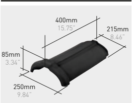
Q01*K | Ridge / Hip klinker
